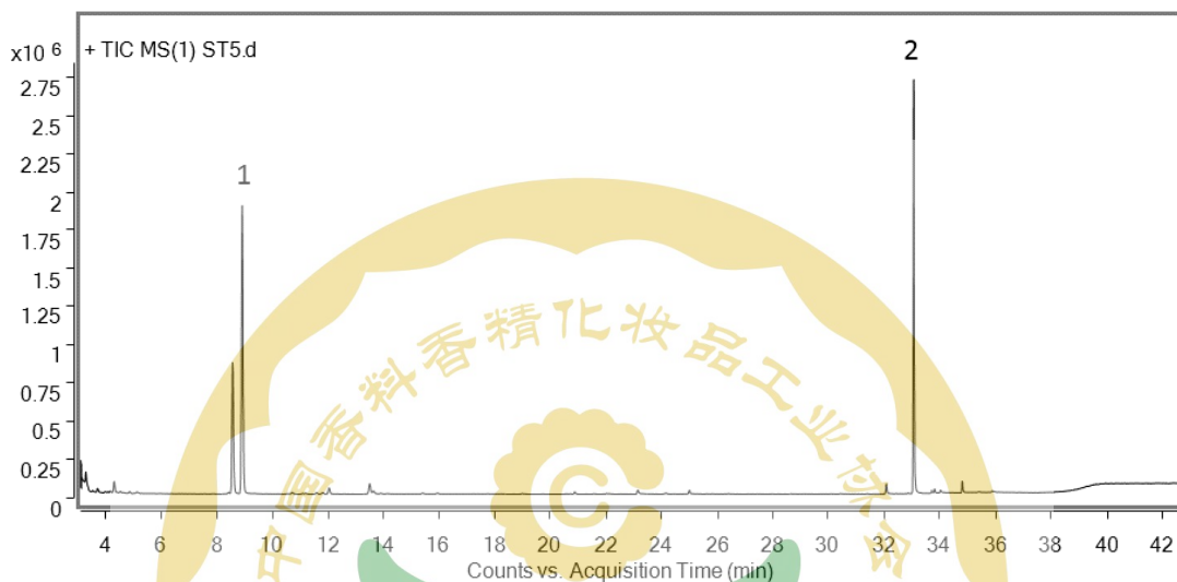
图 B. 1. 1 \beta -罗勒烯和藁本内酯标准品气相色谱-质谱图
