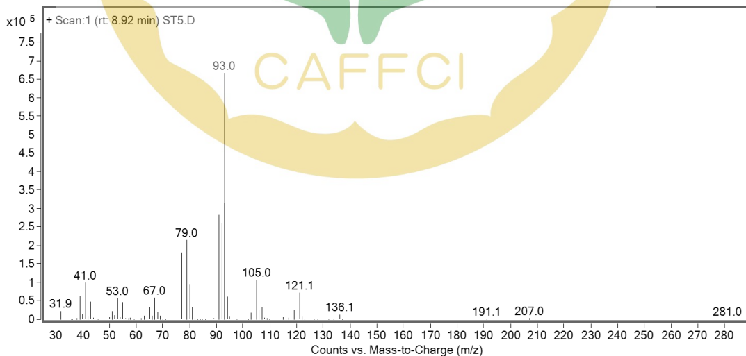
图 B. 1. 2 \beta -罗勒烯标准品质谱图
