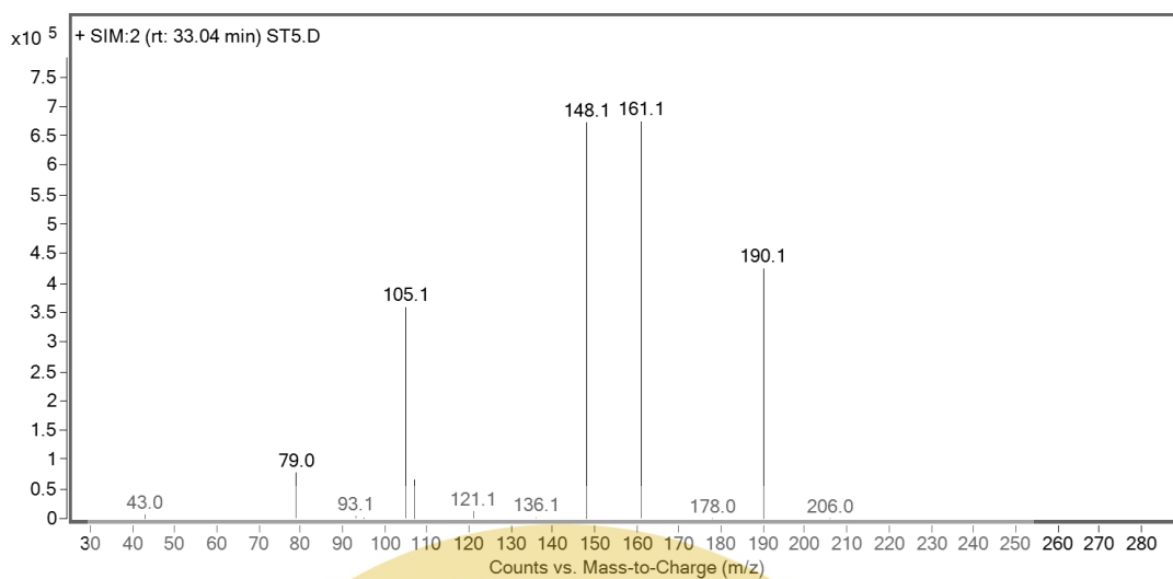
图 B. 1. 3 萘本内酯标准品质谱图
